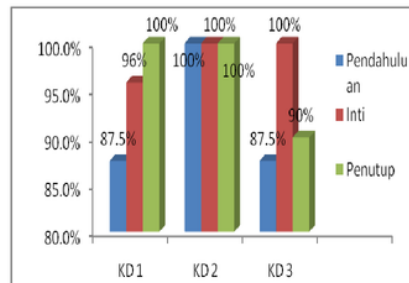
Gambar 1. Histogram keterlaksanaan STAD
