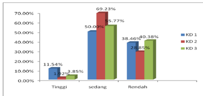
Gambar 3. Histogram pemahaman konsep
