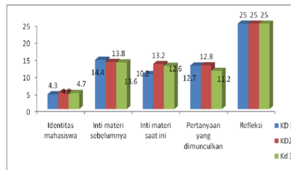
Gambar 2. Histogram hasil penerapan jurnal belajar
